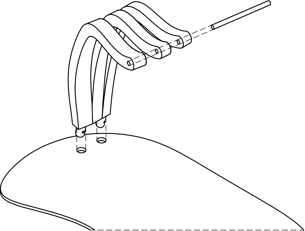
ΛΕΠΤΟΜΕΡΕΙΑ 1
