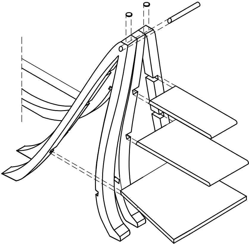
ΛΕΠΤΟΜΕΡΕΙΑ 2
