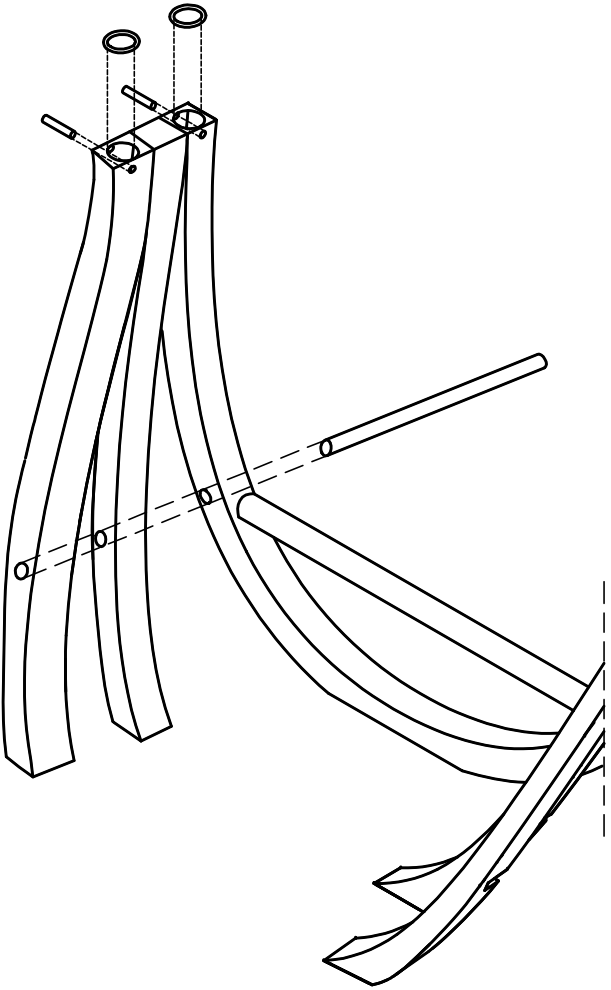
ΛΕΠΤΟΜΕΡΕΙΑ 3
